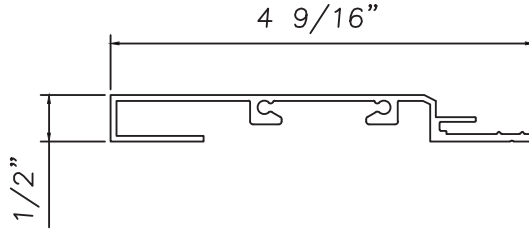
Brighton Panning M20210
