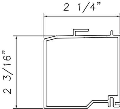
Sill Nose M20557
